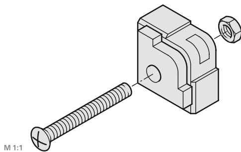
Front-Befestigungselement mit Schraube, für Mauer- und Klingelfronten
