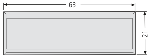
Namensschild 97-9-82174 6,00 € 63 x 21 mm, glasklar, Ausstanzung 60 x 18 mm. Verkauf solange Vorrat reicht.
