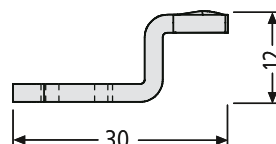
Riegel gekröpft 97-9-00365 2,00 € für Modellgruppe 22 mit Befestigungsfeder
