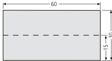
Namensschildeinlage Kunststoff 97-9-87109 0,30 € weiß für Tastenmodule, 60 x 30 x 0,5 mm
