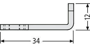
Riegel gekröpft 97-9-00361 4,20 € für verstärkte Türe oder 3-Punkt-Verriegelung mit Befestigungsfeder
