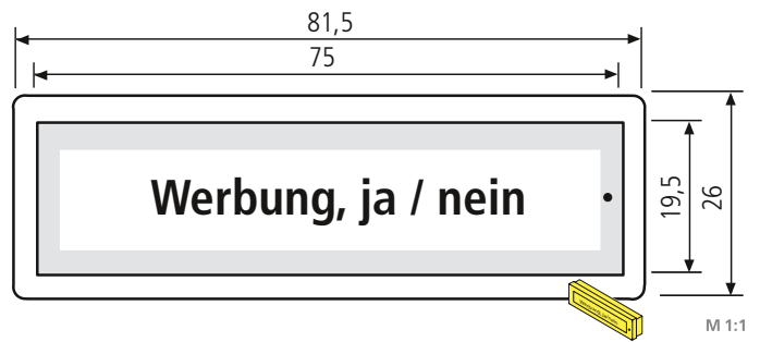
Kunststoff-RSA2 Namensschild 97-9-85368 17,80 € ohne Beleuchtung, mit drehbarer Einlage „Werbung, ja bitte!“ bzw. „Werbung, nein danke!“, mit Montagegehäuse
