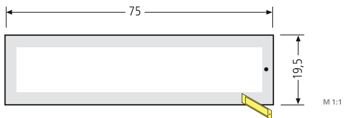
Kunststoff-RSA2 Namensschildabdeckung 97-9-85353 9,10 € für beleuchtetes Schild 97-9-85345, 97-9-85350 Einlage max. 65 x 13,6 x 1 mm
