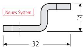
M 1:1 Riegel gekröpft – Auslaufmodell – 97-9-95012 2,00 € für Modellgruppe 22
