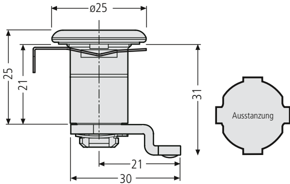
Zylinderschloss ER 97-9-95224 13,20 € Schließung 1-100 inkl. 2 Schlüssel, für Modellgruppe 22 Einbau ab 2006
