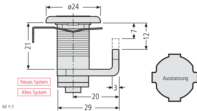
M 1:1 Zylinderschloss 448 97-9-95062 16,00 € Schließung EL 1-200 inkl. 2 Schlüssel, mit zwei Riegeln, Einbau seit 1993
