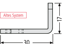
Riegel gekröpft 97-9-00364 2,00 € für altes System mit Befestigungsfeder (Standard-Briefkästen)
