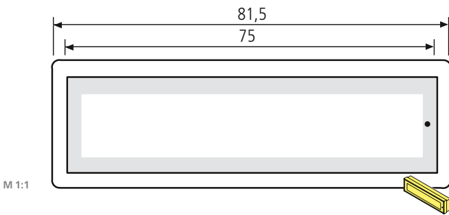
Kunststoff-RSA2 Namensschild 97-9-85356 15,80 € ohne Beleuchtung, mit Montagegehäuse, Einlage max. 65 x 13,6 x 1 mm
