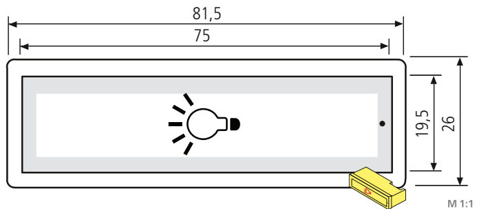
Kunststoff-RSA2 Lichtschild 97-9-85350 23,70 € mit Lichtsymbol-Einlage, mit LED-Beleuchtung , Anschluss 12 – 24 V, 0,12 Watt AC/DC, mit Montagegehäuse
