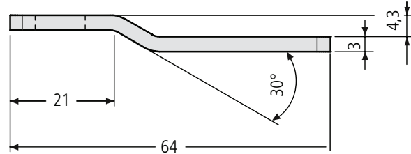
M 1:1 Riegel für Renz-Depotbox 97-9-00437 4,20 € für „Schwere Baureihe“
