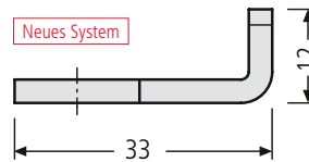
M 1:1 Riegel gekröpft – Auslaufmodell – 97-9-95011 2,00 € für verstärkte Tür
