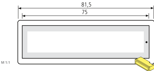
Kunststoff-RSA2 Namensschild für RSA2 -Klingel 97-9-85345 22,40 € mit LED-Beleuchtung , Anschluss 12 – 24 V, 0,12 Watt AC/DC mit Montagegehäuse, Einlage max. 65 x 13,6 x 1 mm
