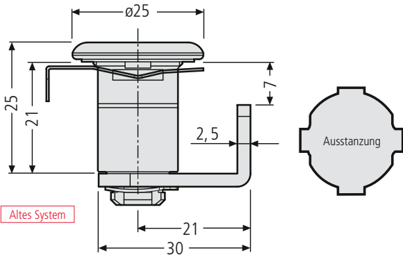
Zylinderschloss ER 97-9-95223 13,20 € Schließung 1-50 inkl. 2 Schlüssel, Einbau ab 2006
