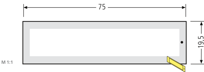
Kunststoff-RSA2 Namensschildabdeckung 97-9-85357 8,60 € für unbeleuchtetes Schild 97-9-85356, 97-9-85368, Einlage max. 65 x 13,6 x 1 mm
