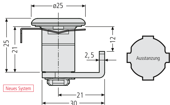
Zylinderschloss ER 97-9-95221 13,20 € Schließung 1-400 inkl. 2 Schlüssel, Einbau ab 2006
