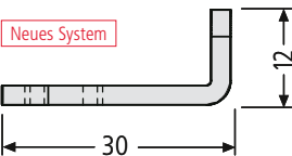
Riegel gekröpft 97-9-00363 2,00 € für neues System mit Befestigungsfeder (Standard-Briefkästen)
