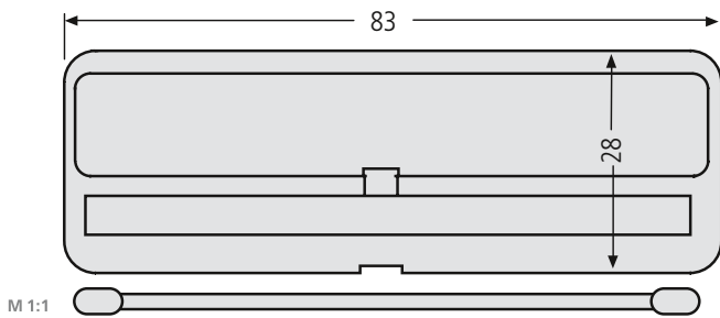
Klappenhalter 97-9-82193 5,80 € mit Torsionfeder, 83 x 28 mm, Verkauf solange Vorrat reicht.
