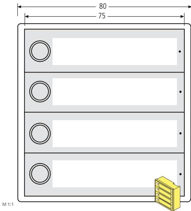
Kunststoff-RSA2-kompakt-Block, 4 Namensschilder 97-9-85329 166,20 € – Einbau seit 2009 – ohne Gravur, mit Montagegehäuse, Einlage max. 59 x 13,6 x 1 mm, Anschluss 12 – 24 V, inkl. LED-Beleuchtungsringen je 0,12 Watt AC/DC
