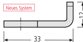
M 1:1 Riegel gekröpft – Auslaufmodell – 97-9-95014 4,20 € für 3-Punkt-Verriegelung Serienkästen
