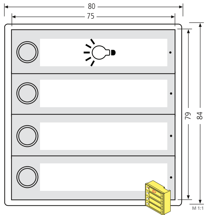
Kunststoff-RSA2-kompakt-Block, 3 Namensschilder + 1 Lichtschild 97-9-85331 167,50 € – Einbau seit 2009 – ohne Gravur, mit Montagegehäuse, Einlage max. 59 x 13,6 x 1 mm, Anschluss 12 – 24 V, inkl. LED-Beleuchtungsringen je 0,12 Watt AC/DC
